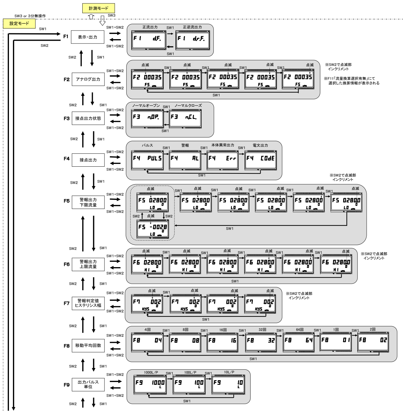
図 2-1 設定モードの表示切替フロー (B, D) (1/2)
