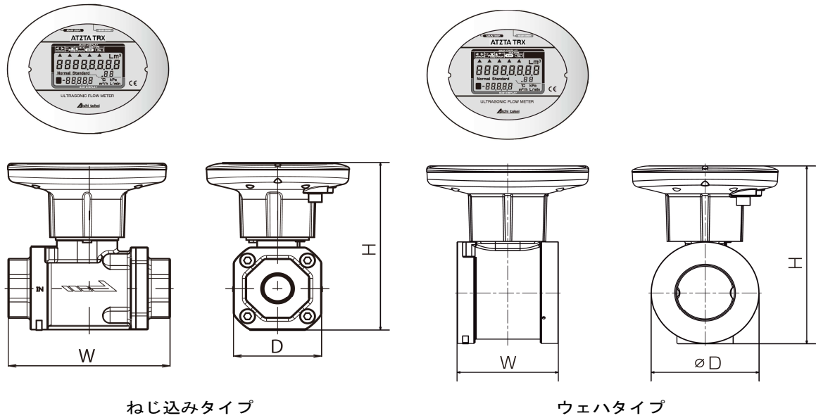
図 10-1 外形図
